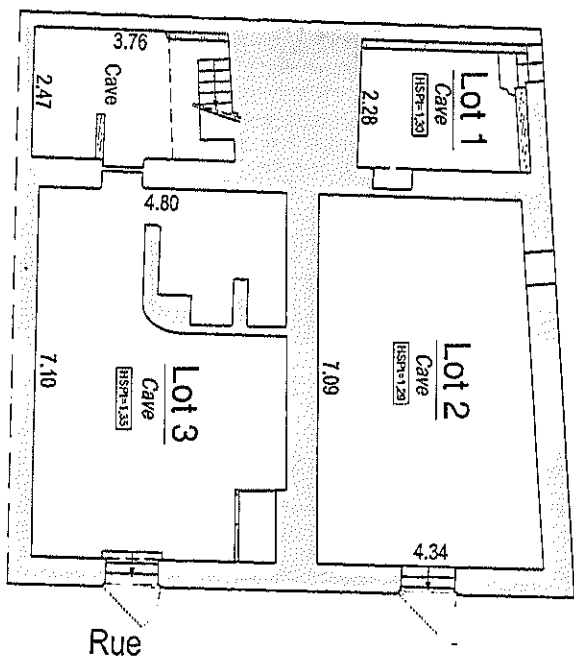
Sous-sol
